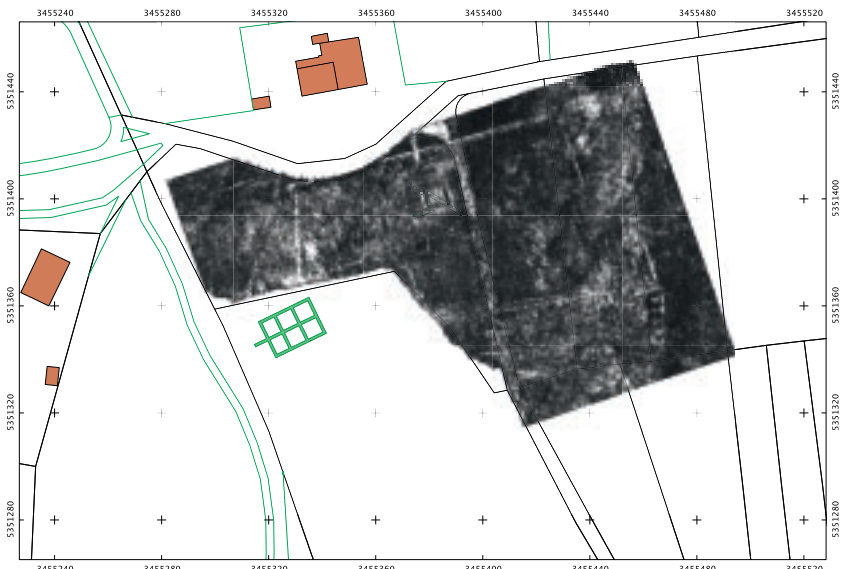
7 Geophysikalische Messungen im Januar 2013 durch Harald von der Osten-Woldenburg.
